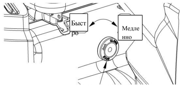
Ручка регулировки скорости опускания
